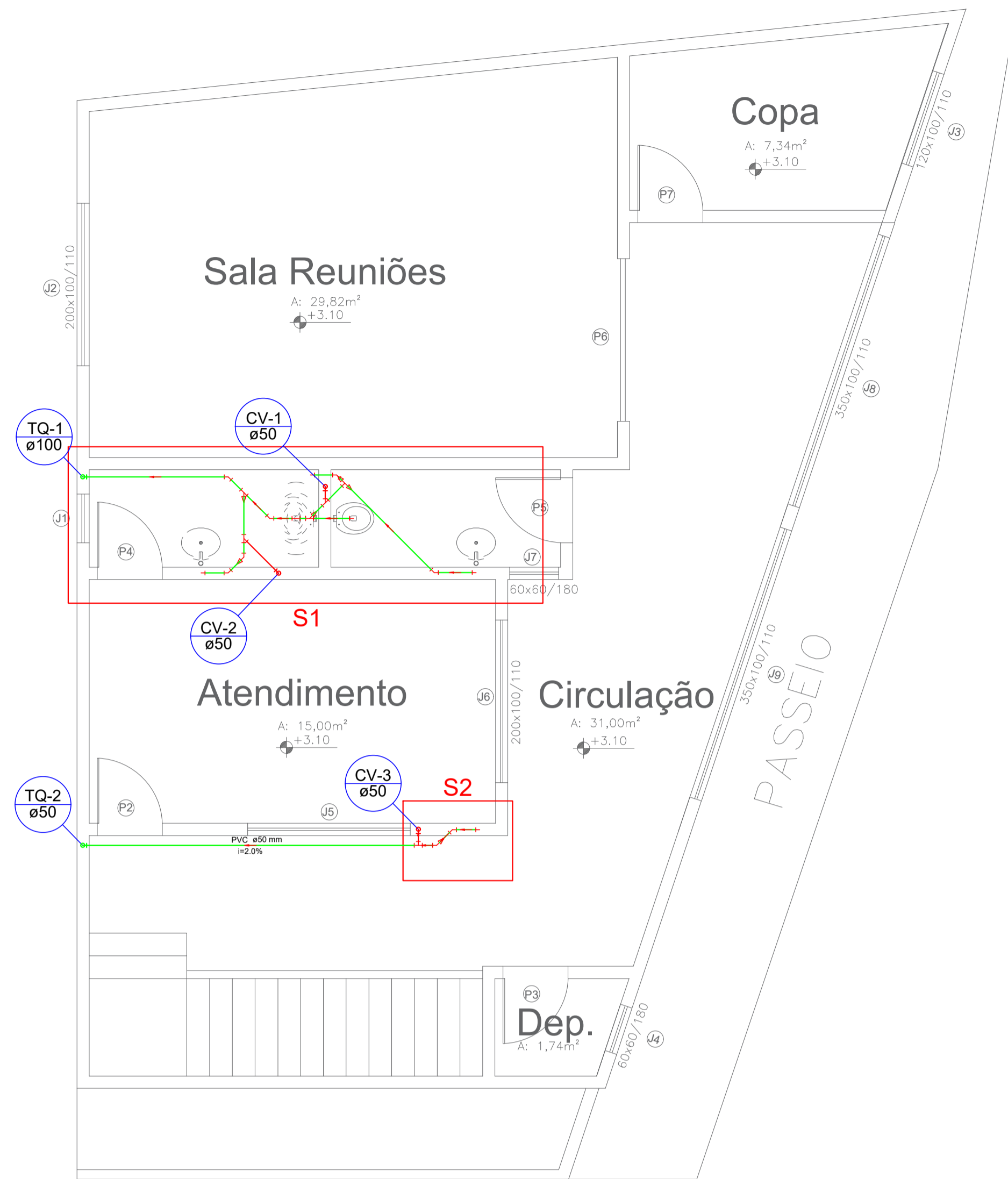
PLANTA BAIXA 1º ANDAR - ÁREA 109,57 m² ESCALA 1 : 75
