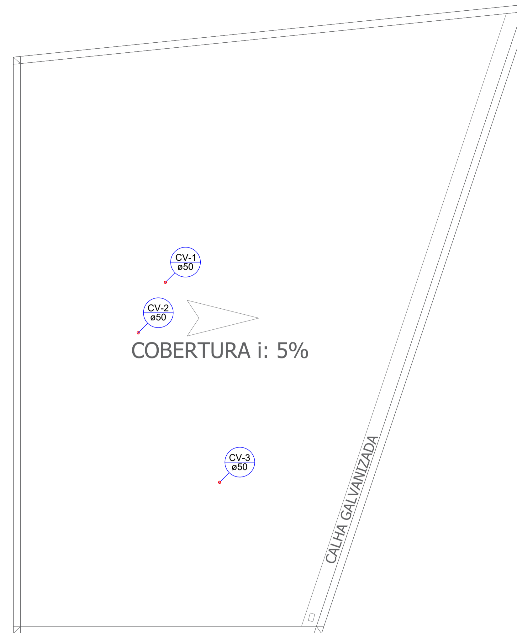
DIAGRAMA DE COBERTURA ESCALA 1 : 50
