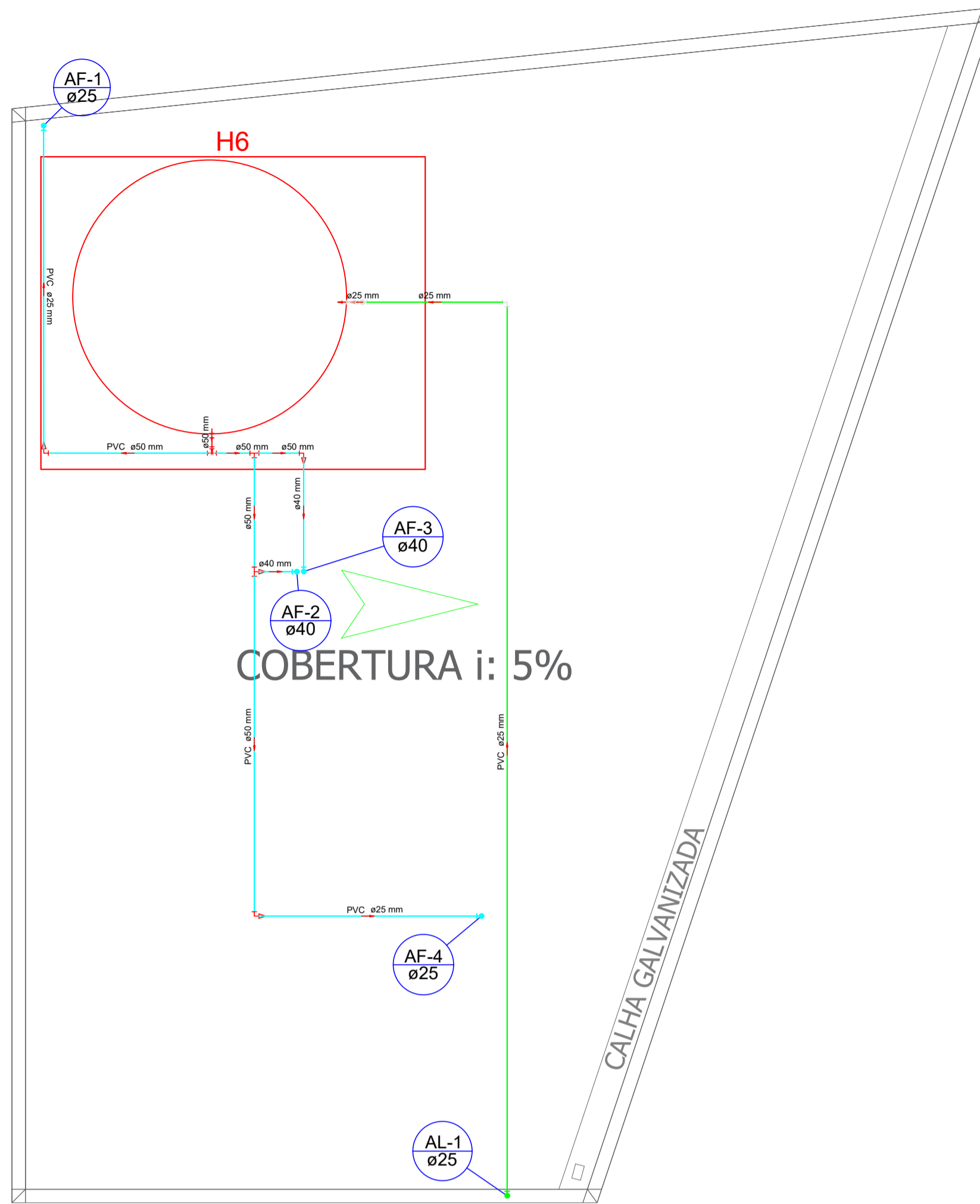
COBERTURA ESCALA 1 : 50
