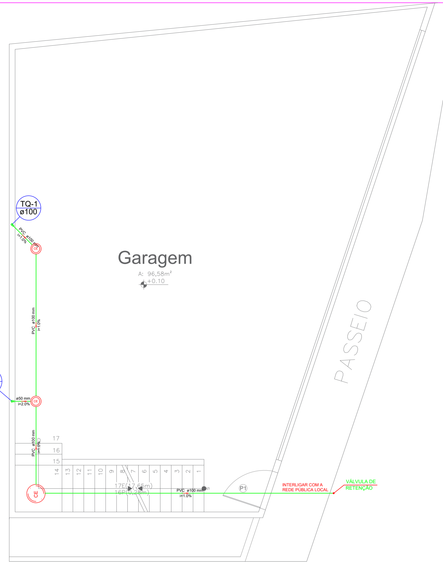
PLANTA BAIXA TÉRREO - ÁREA 109,57 m 2 ESCALA 1 : 75
